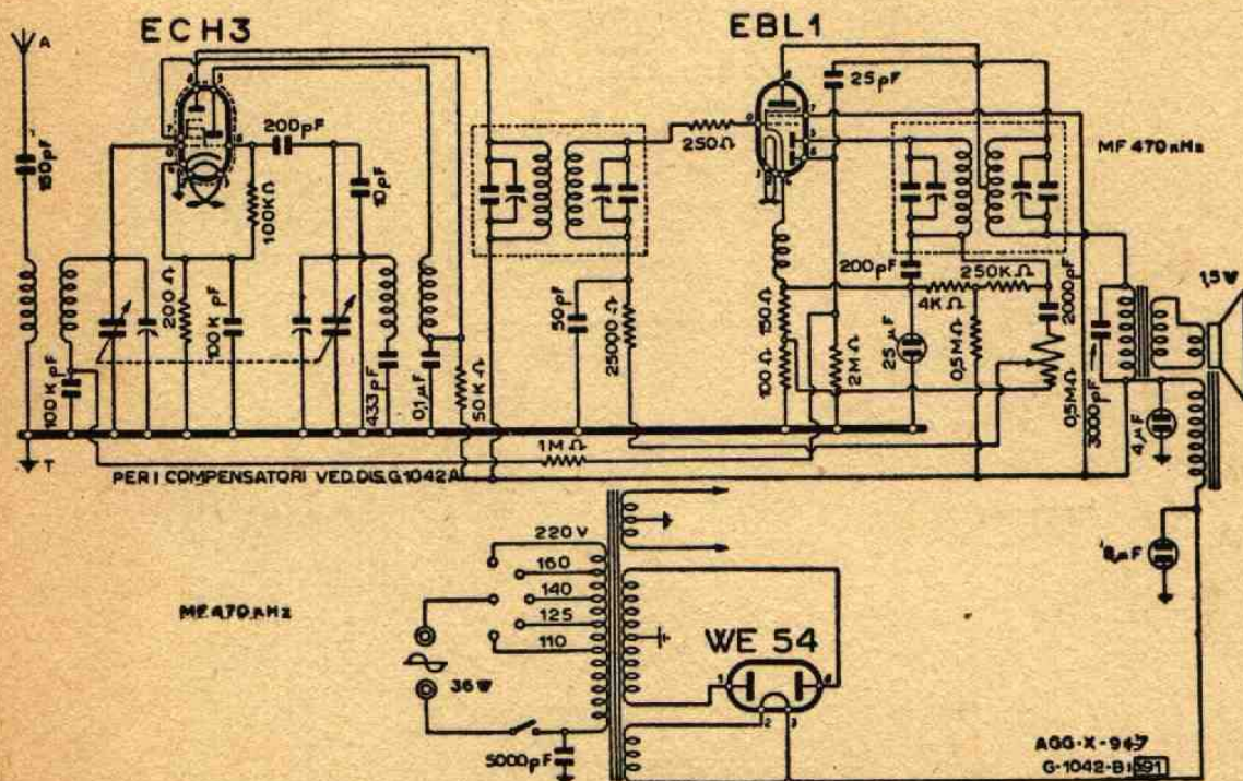
Lo schema elettrico del Phonola 301/2
