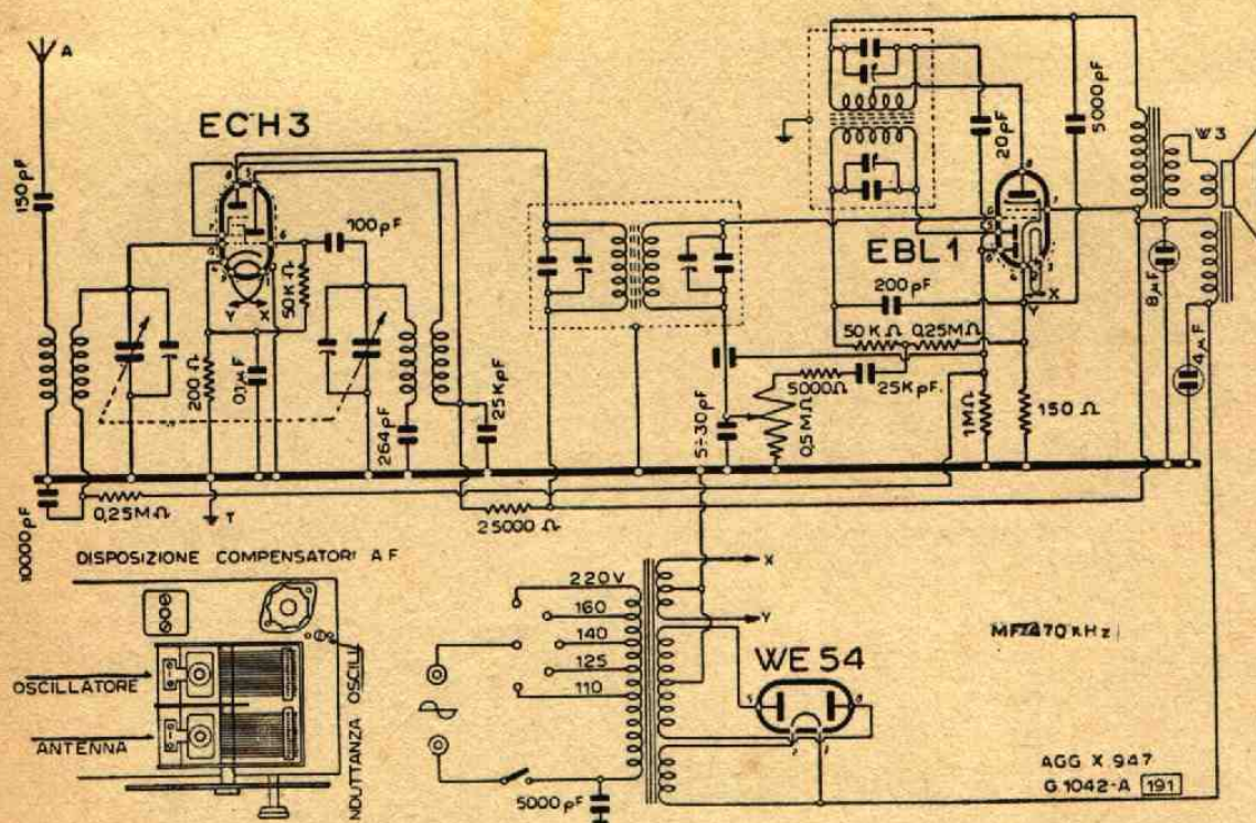
Lo schema elettrico del Phonola 301
